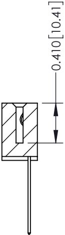
SECTION A-A
