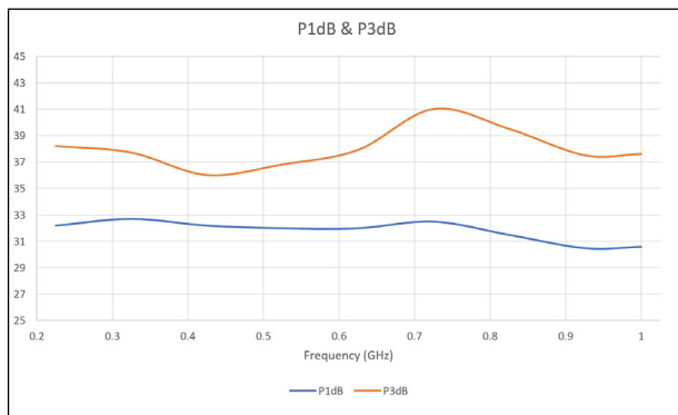
P1dB & P3dB
