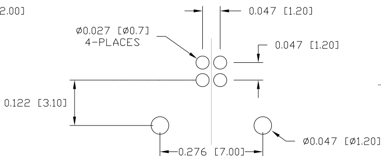
P.C.B LAYOUT
