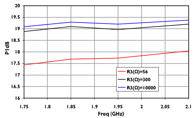
P1dB
