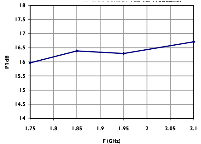
P1dB
